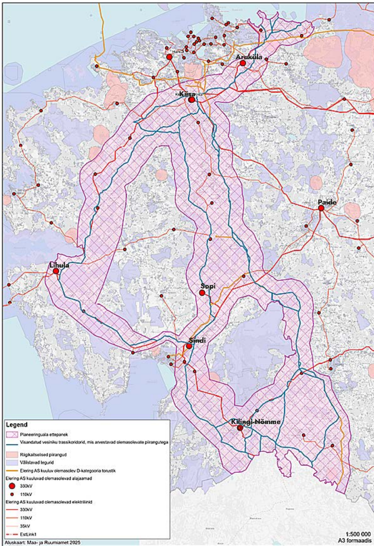
Vesinikutaristu võimalikud trassikoridorid Eestis.
