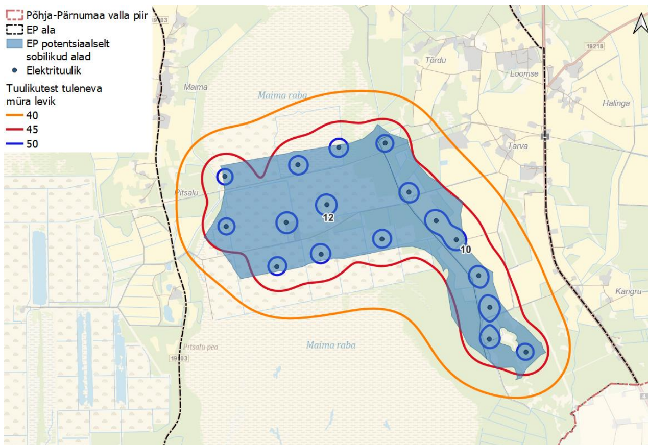
Skeem 82. Potentsiaalselt sobilike alade 10 ja 12 müra leviku modelleerimise tulemused tuuleparkide maksimaalse arenduse korral.
