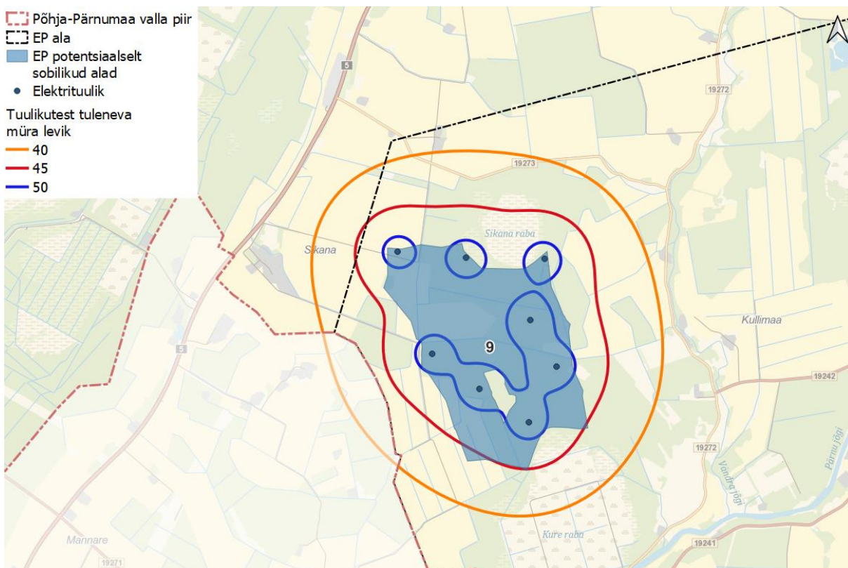
Skeem 81. Potentsiaalselt sobiliku ala 9 müra leviku modelleerimise tulemused tuulepargi maksimaalse arenduse korral.
