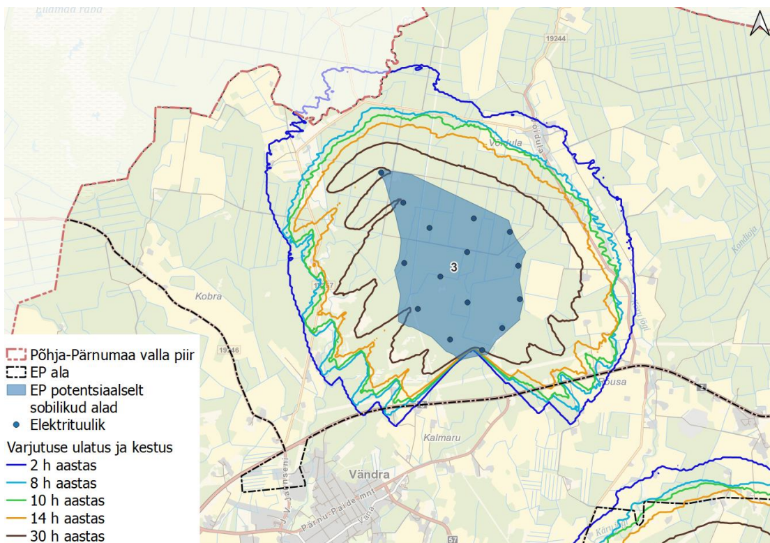
Skeem 88. Potentsiaalselt sobiliku ala 3 tegelikult võimalik varjutuskaart (ilma taimkatteta) eriplaneeringu alal 1.
