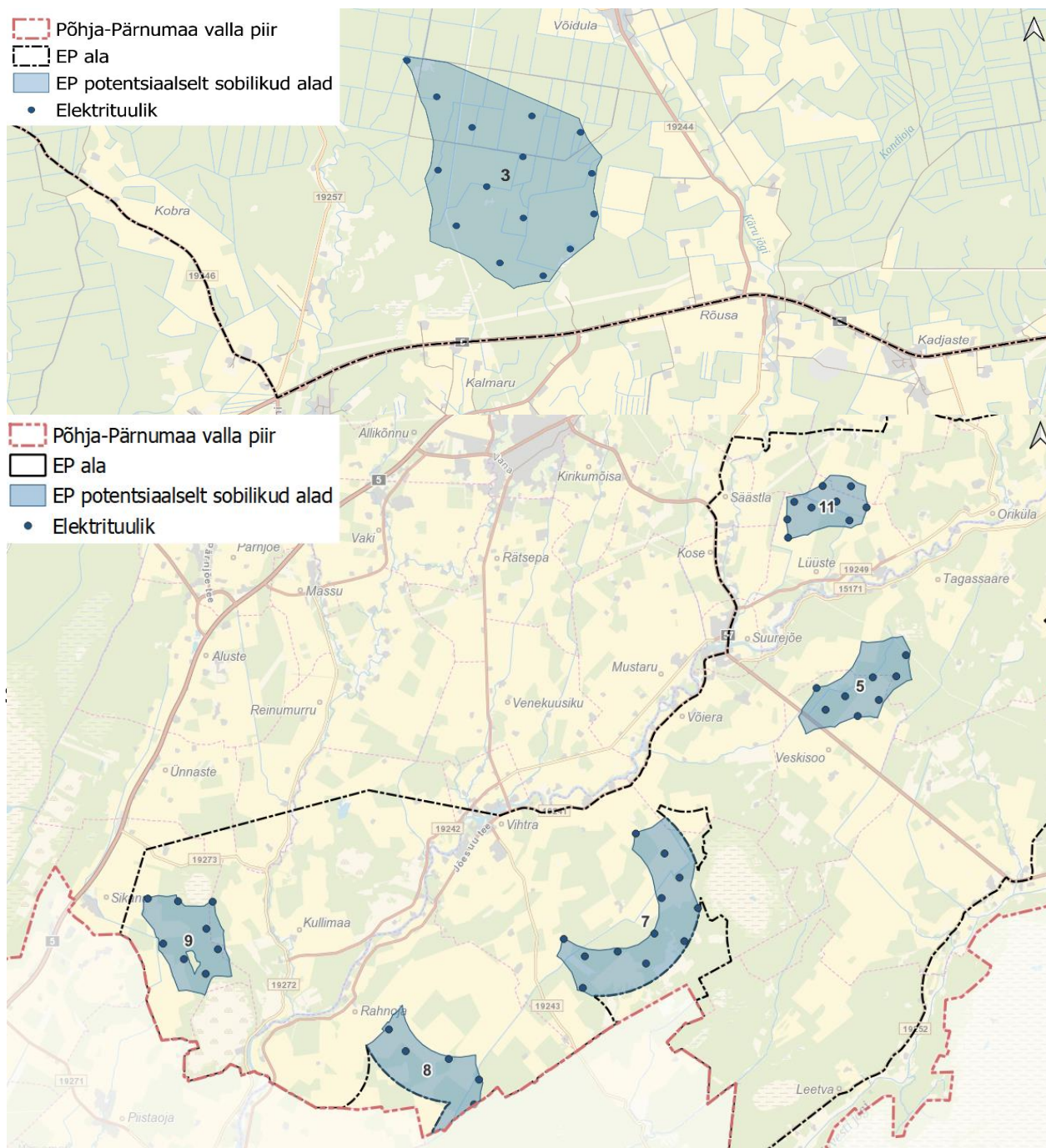
Skeem 74. Tuulikute arv ja võimalik paiknemine eriplaneeringu potentsiaalselt sobilikel aladel.
