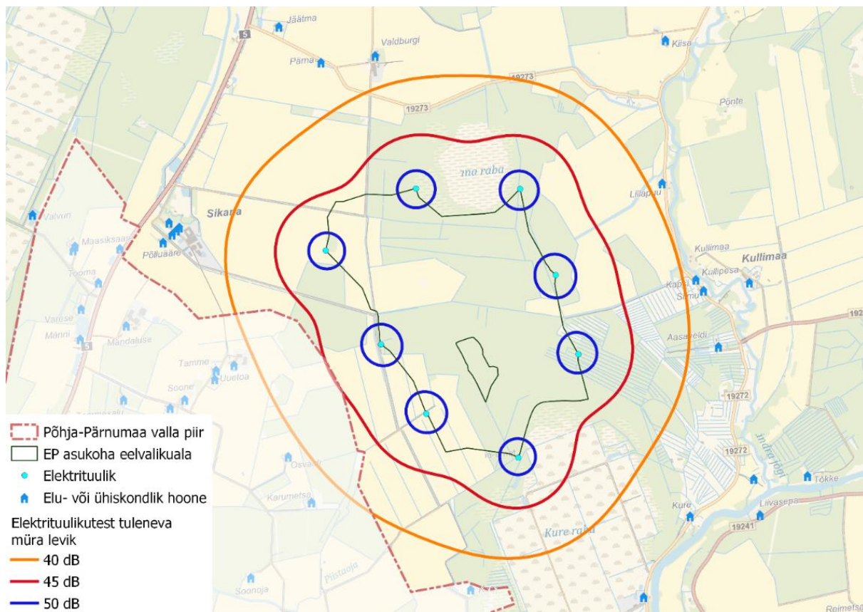
Skeem 118. Eelvalikuala nr 9 müra modelleerimistulemused halvima stsenaariumi korral.
