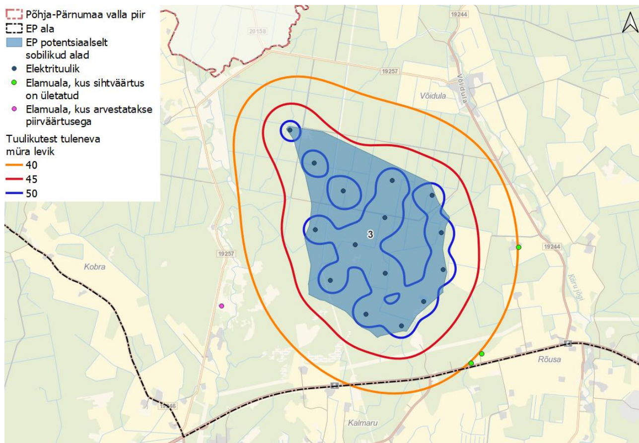
Skeem 77. Potentsiaalselt sobiliku ala 3 müra leviku modelleerimise tulemused tuulepargi maksimaalse arenduse korral.
