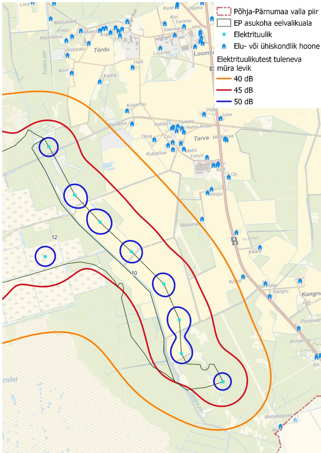
Skeem 115. Eelvalikuala nr 10 müra modelleerimistulemused halvima stsenaariumi korral, pärast ala piiride korrigeerimist.
