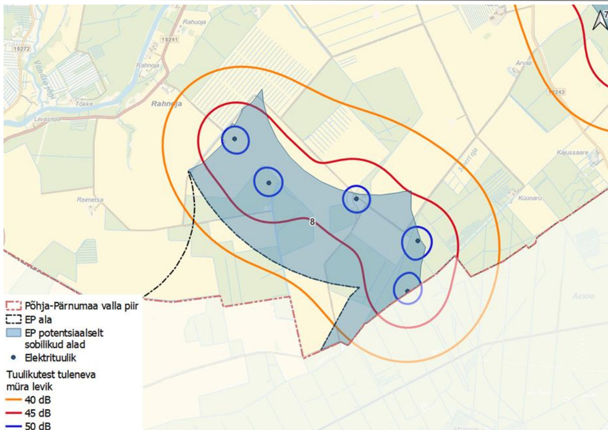
Skeem 80. Potentsiaalselt sobiliku ala 8 müra leviku modelleerimise tulemused tuulepargi maksimaalse arenduse korral.
