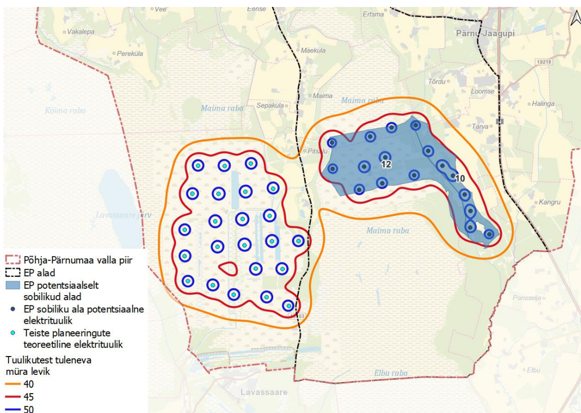
Skeem 85. Põhja-Pärnumaa eriplaneeringu potentsiaalselt sobilike alade ja teiste planeeringute tuulepargialade omavahelise kumulatiivse müra modelleeringu tulemused.
