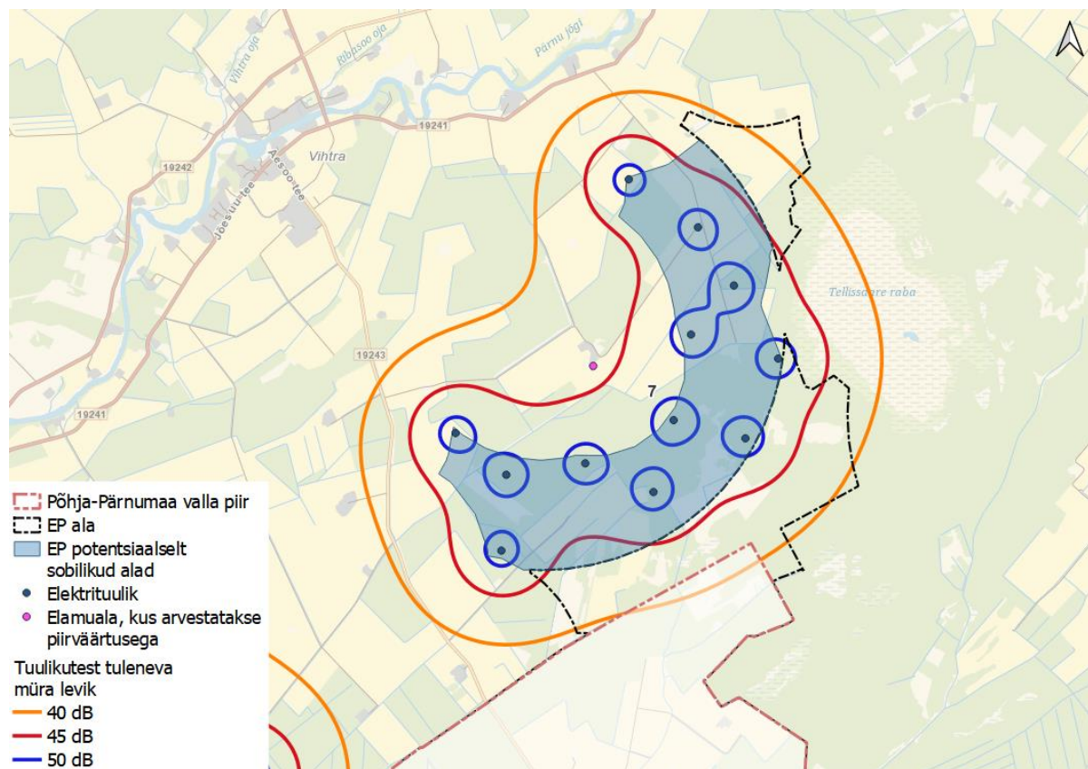
Skeem 79. Potentsiaalselt sobiliku ala 7 müra leviku modelleerimise tulemused tuulepargi maksimaalse arenduse korral.
