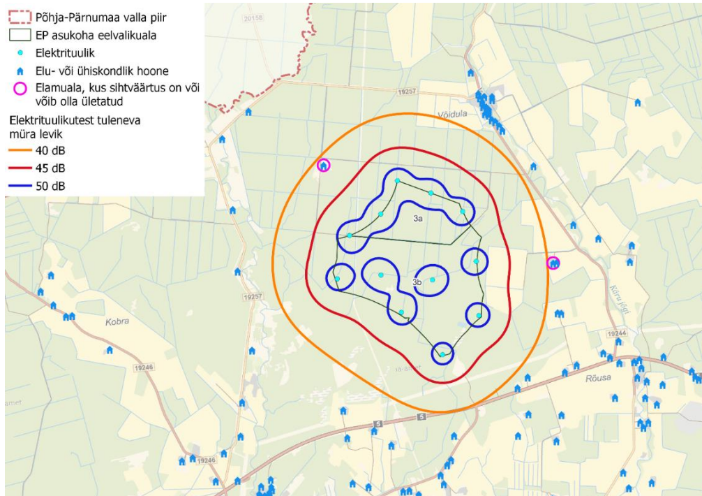
Skeem 116. Eelvalikuala nr 3a müra modelleerimistulemused halvima stsenaariumi korral. Arvestatud on ka eelvalikuala nr 3b kumulatiivset mõju.
