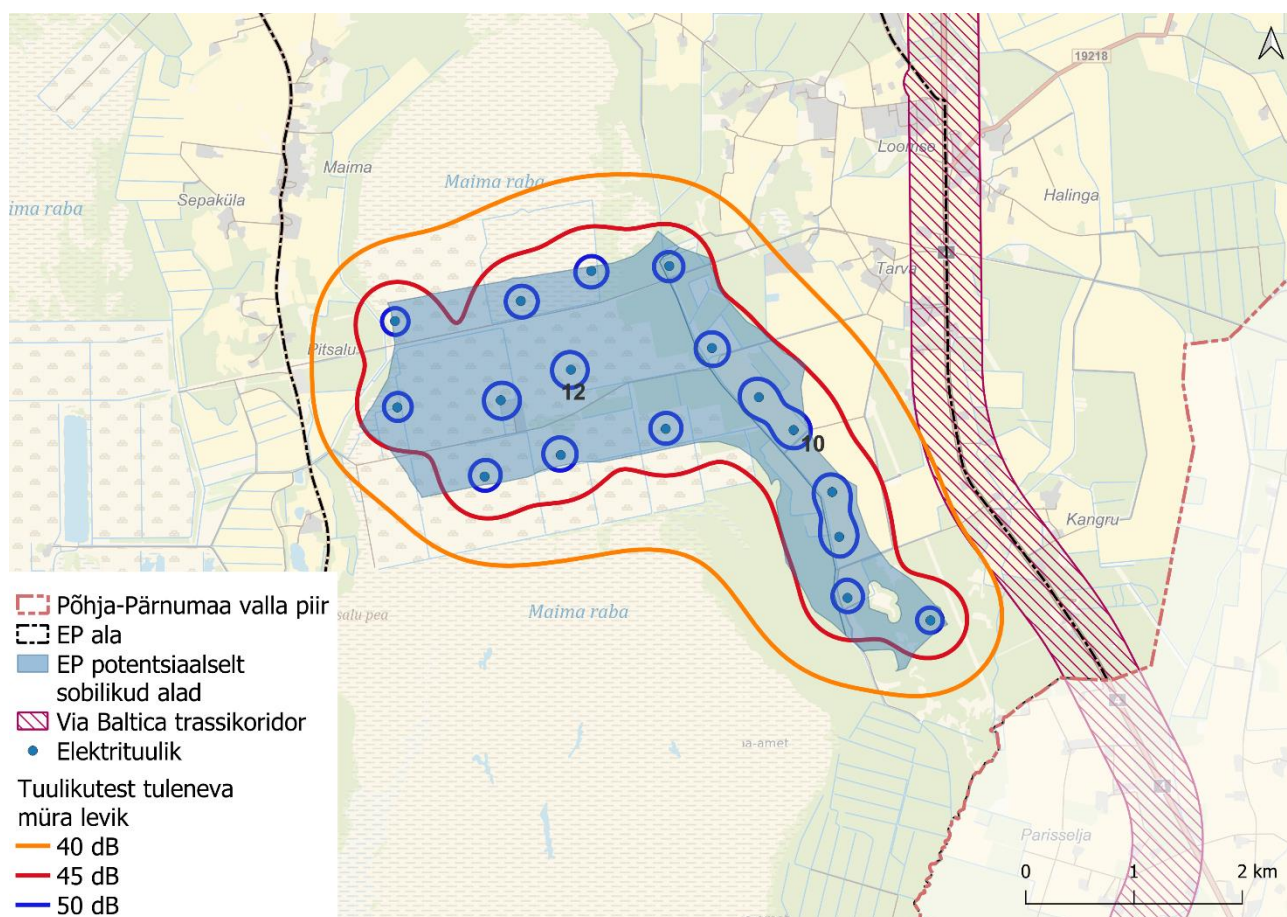
Skeem 86. Via Baltica trassikoridori paiknemine ning eriplaneeringu potentsiaalse ala 10 ja 12 müra modelleerimistulemused.
