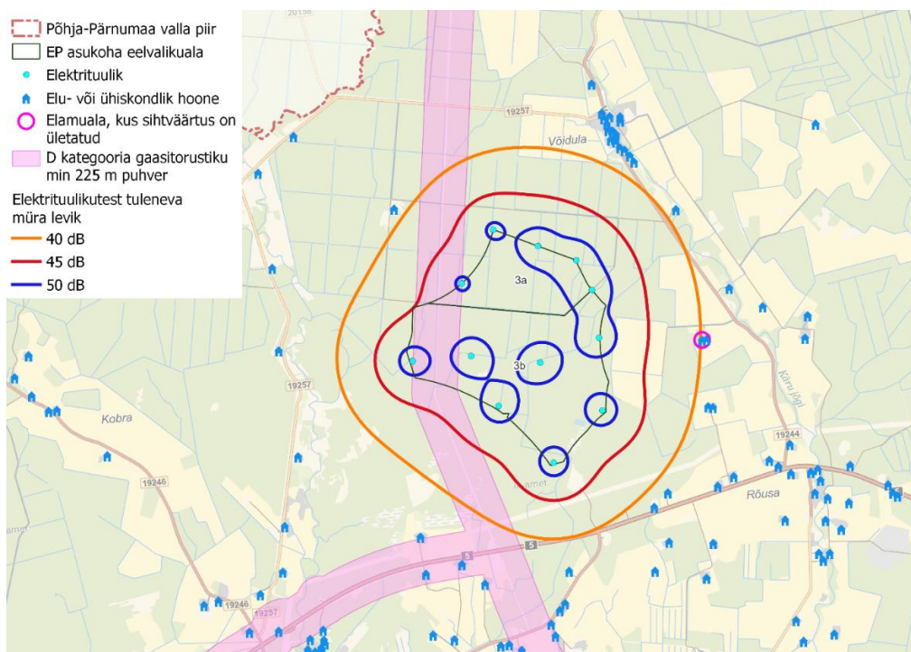
Skeem 117. Eelvalikuala nr 3a müra modelleerimistulemused halvima stsenaariumi korral, pärast tingimuste muutmist 37
