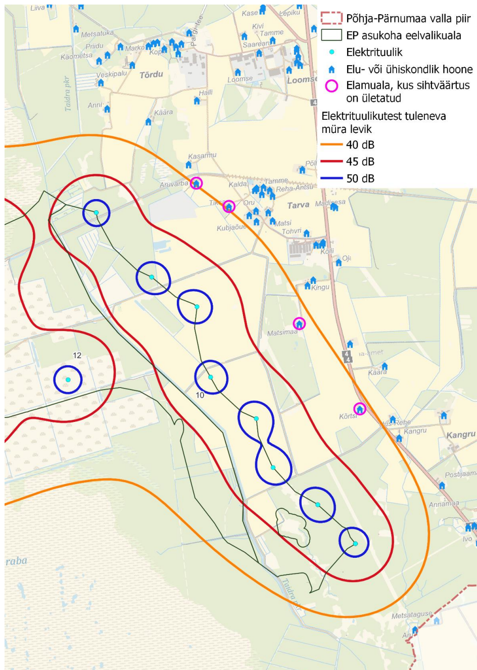
Skeem 114. Eelvalikuala nr 10 müra modelleerimistulemused halvima stsenaariumi korral. Arvestatud on ka eelvalikuala nr 12 kumulatiivset mõju.
